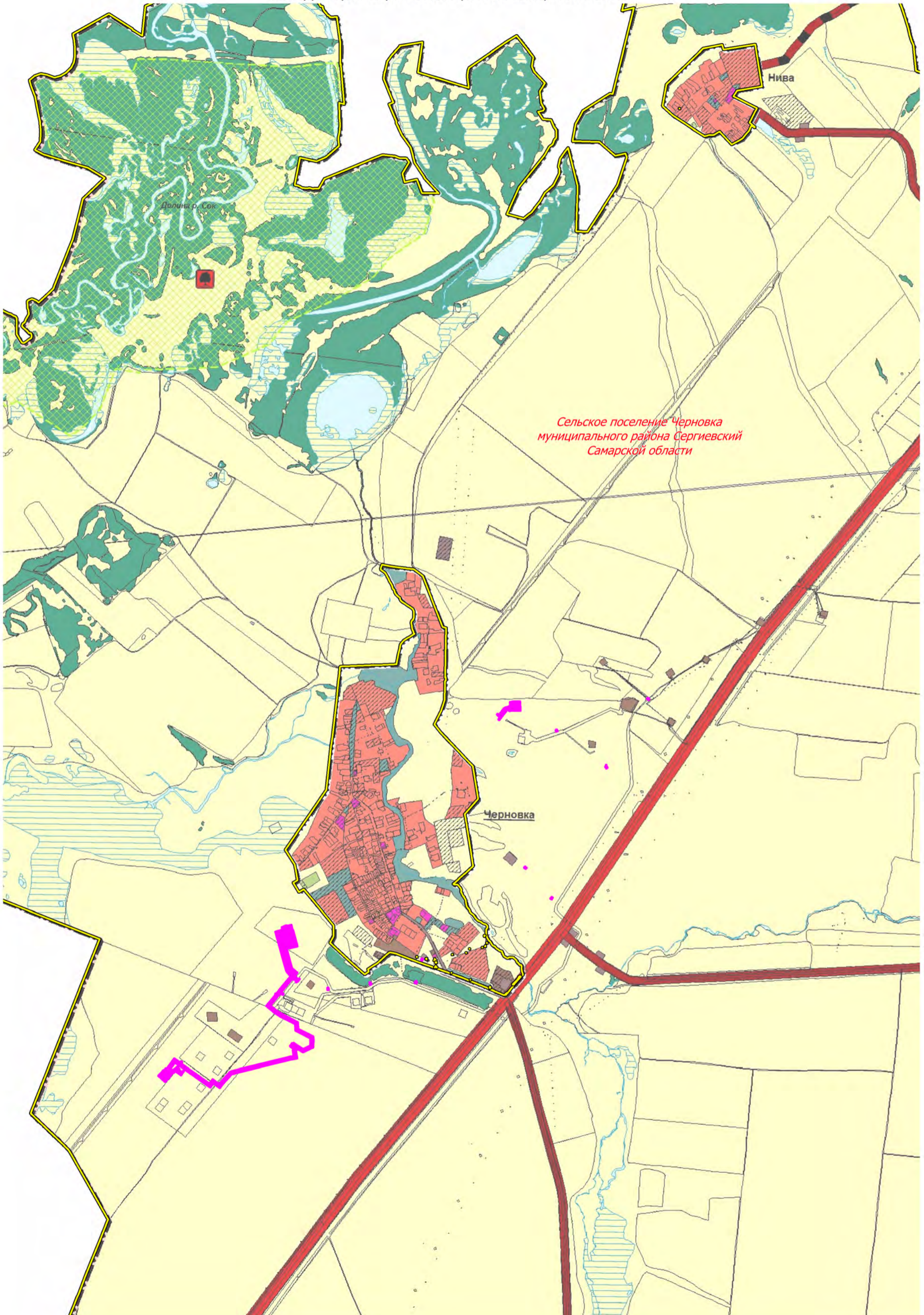
Схема границ разработки документации по планировке территории объекта 8820П "Сбор нефти и газа со скважин №№ 156, 254, 255 и электроснабжение скважин №№ 251, 252 Южно-Орловского месторождения" на территории Сергиевского района Самарской области
